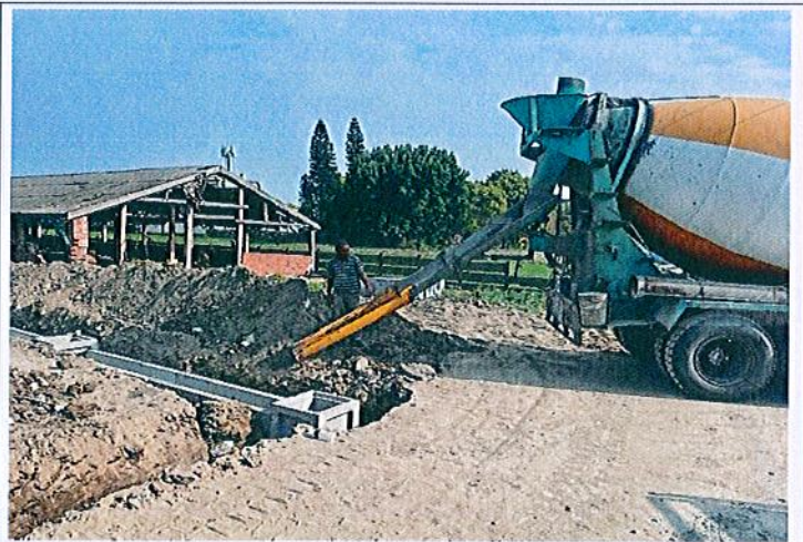
水溝埋設工程、1樓水電配管
